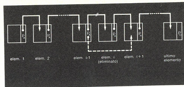
Fig. 5 - Eliminazione di un elemento da una catena unidirezionale: P_A = Puntatore avanti, P_O = Puntatore nullo.
