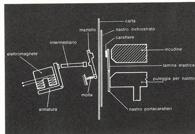
Fig. 11 - Stampante a nastro: meccanismo di stampa.
