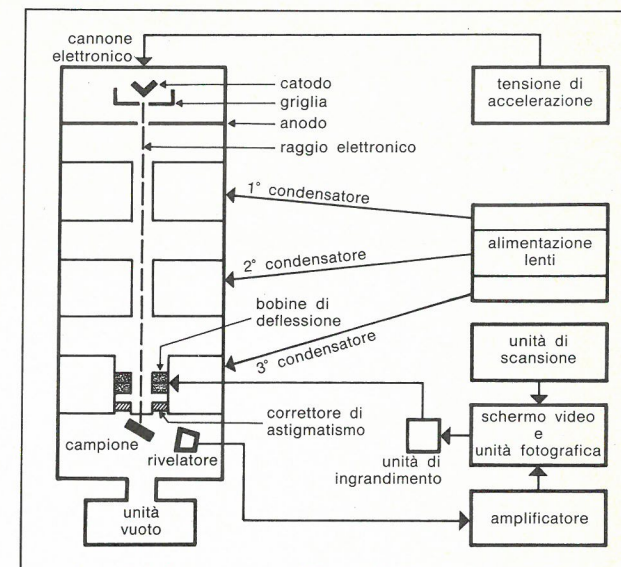
Fig. 1 - Componenti principali di un microscopio elettronico a scansione.
