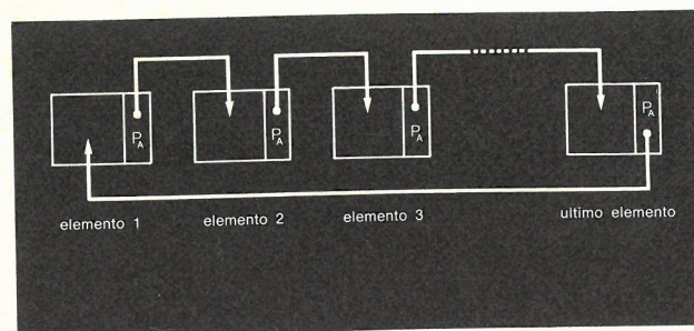
Fig. 4 Schema di catena circolare (unidirezionale): P_A = Puntatore avanti.
