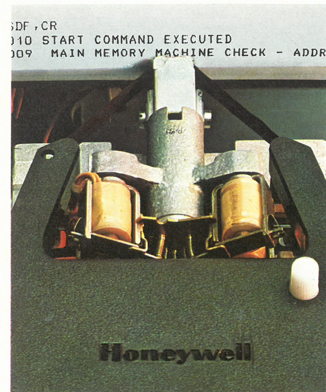
Fig. 18 - Le fotografie mostrano la testina di una moderna stampante seriale a matrice di alte prestazioni. (Progetto e fabbricazione della Honeywell Information Systems Italia).
