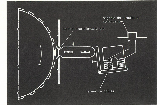
Fig. 7 - Stampante a tamburo: a) meccanismo a riposo; b) meccanismo in lavoro.
