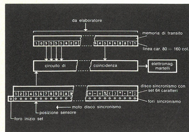
Fig. 5 - Schema di funzionamento di stampante a tamburo.
