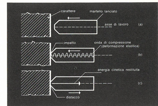
Fig. 8 - Stampa « al volo » con controllo dell'energia cinetica.
