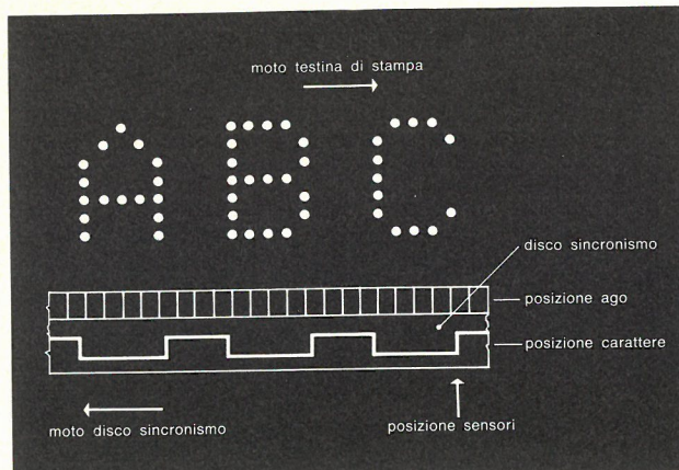
Fig. 16 - Principio di stampa a matrice di punti.
