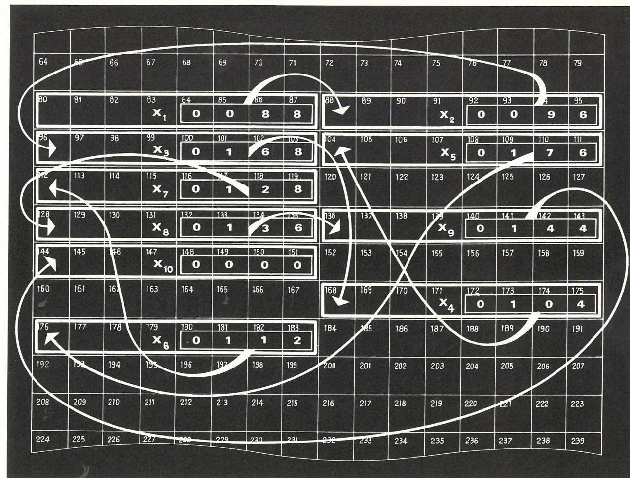
Fig. 2 - Una struttura concatenata
