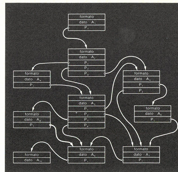
Fig. 7 - Schema di plesso: A_1, A_2, \dots, A_{10} = Dati associati ai nodi del grafo rappresentato; P_1, P_2, P_3, P_4 = Puntatori.
