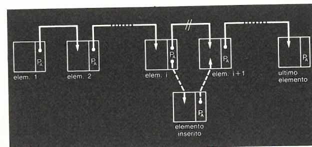
Fig. 6 - Inserimento di un elemento in una catena (unidirezionale): P_A = Puntatore avanti, P_O = Puntatore nullo.
