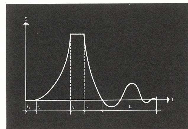
Fig. 19 - Diagramma di moto degli aghi in una stampante seriale a matrice.
