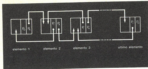
Fig. 3 - Schema di catena bidirezionale: P_A = Puntatore avanti (all'elemento successivo), P_I = Puntatore indietro (all'elemento precedente), P_O = Puntatore nullo (fine catena).
