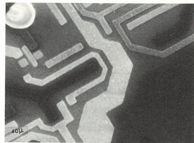
Fig. 3 - Particolare di un circuito integrato osservato durante il suo funzionamento. Le zone scure denotano un potenziale positivo, quelle chiare sono a potenziale di massa.
