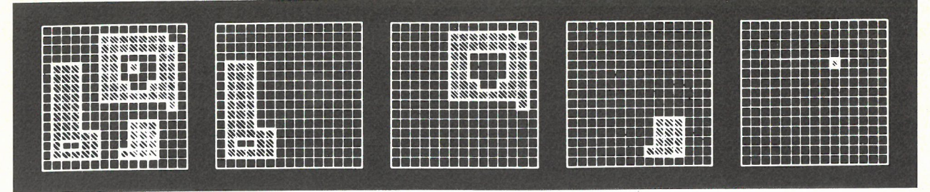
Fig. 5 - Estrazione delle componenti connesse in una immagine binaria [24].
