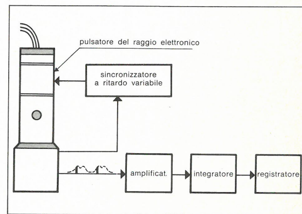
Fig. 2 - Principio di funzionamento di un sistema stroboscopico in microscopia elettronica a scansione.
