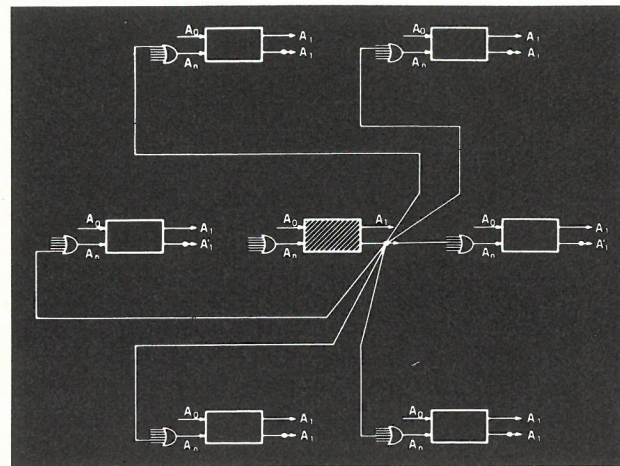
Fig. 6 - Elemento di memoria e logica di una macchina parallela di tipo CLIP [23].
