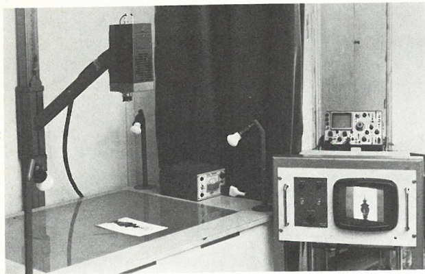
Fig. 2 - Sistema di acquisizione e digitalizzazione mediante telecamera (VIP - Video Input Processor).
